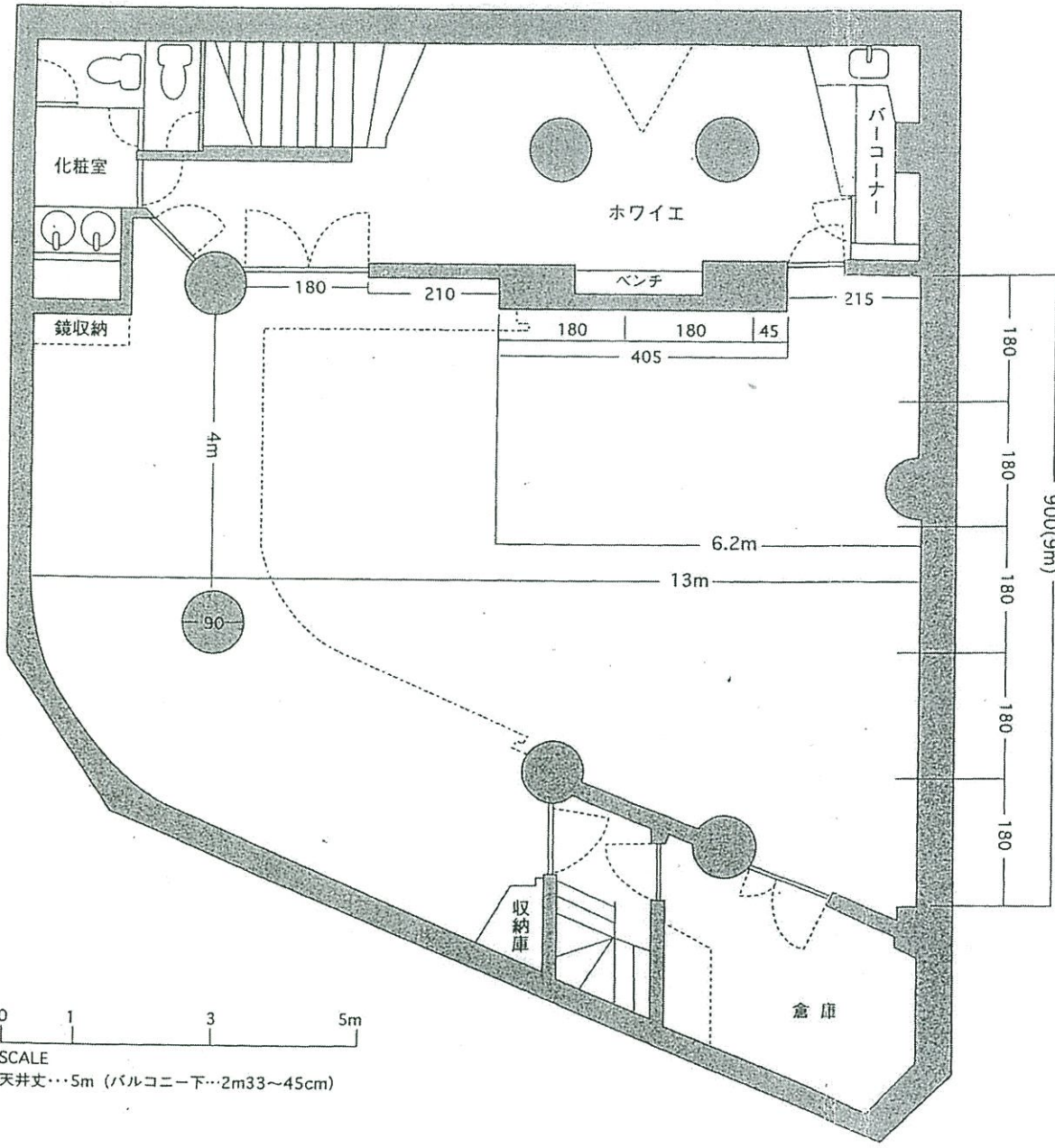
セッションハウス B1 平面図
